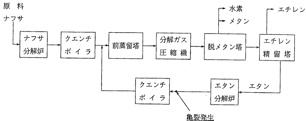
プロセスのブロック線図
