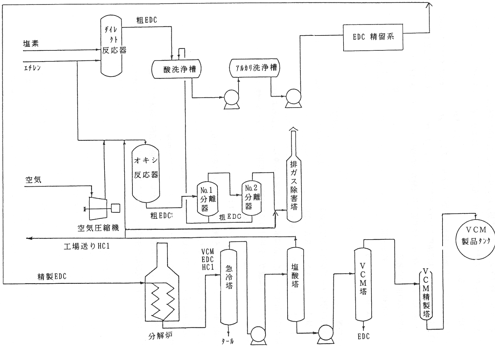
塩化ビニールモノマー (VCM) 製造工程図
