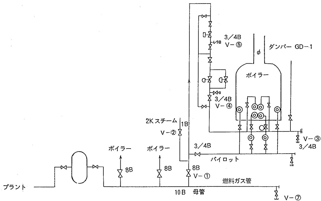
発電用水管式ボイラー配管フロー図
