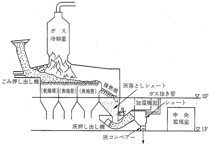
焼却炉の概略図と爆発位置
