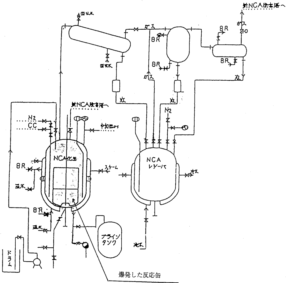
ベンジルクロロホーマートプロセスライン図
