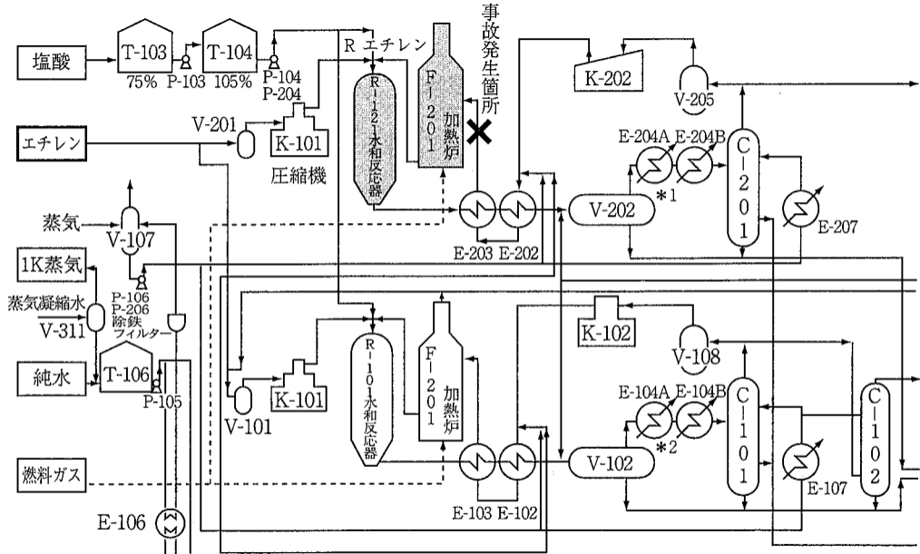
エタノールプラント フローダイアグラム
